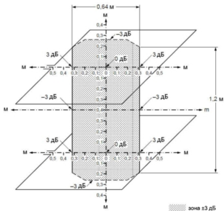
Рисунок В.5 – Зона ±3 дБ магнитного поля, создаваемого двумя индукционными катушками квадратной формы (с длиной стороны 1 м), разнесенными на расстояние 0,8 м, в центральной ортогональной плоскости (компонента, перпендикулярная плоскости катушки)
