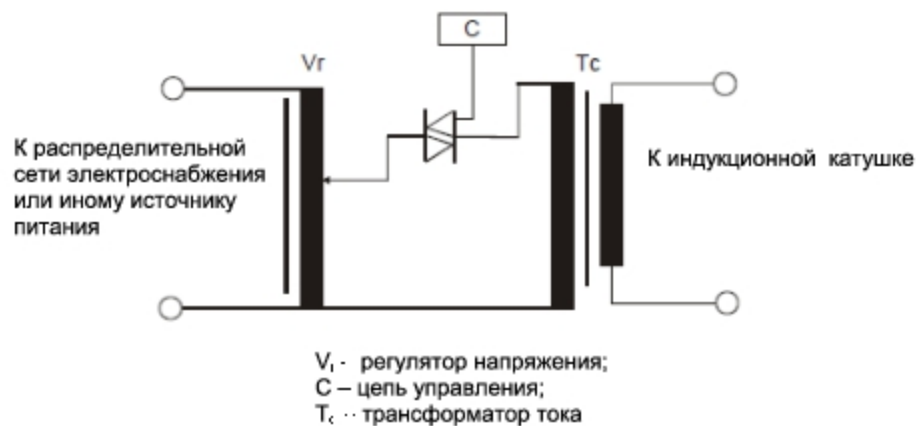
Рисунок 2 – Схема испытательного генератора магнитного поля промышленной частоты
