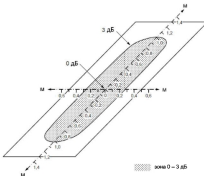
Рисунок В.6 – Зона ±3 дБ магнитного поля, создаваемого индукционной катушкой прямоугольной формы (с размерами сторон 1 × 2,6 м) в плоскости катушки
